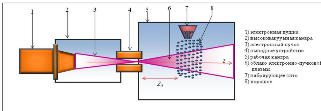
Рис. 1. Схематичное изображение установки для компьютерного моделирования ЭПП
